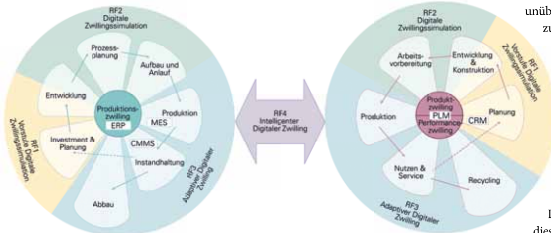
Verknüpftes Wertstromzyklusmodell im Reifegradmodell. (Grafik: FHNW)
